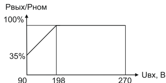
Рисунок 1. Зависимость выходной мощности от входного напряжения, где U_{вх} – входное напряжение, R_{вых} – выходная мощность, R_{ном} – номинальная (паспортная) выходная мощность.
