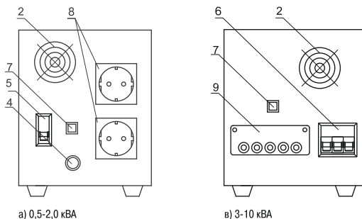
Рисунок 3. Переносной стабилизатор, вид сзади.
