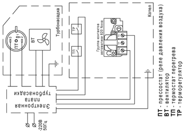
Схема подключения турбонасадки "Лемакс Comfort SE" к энергонезависимому котлу с автоматикой SIT 820 Nova
